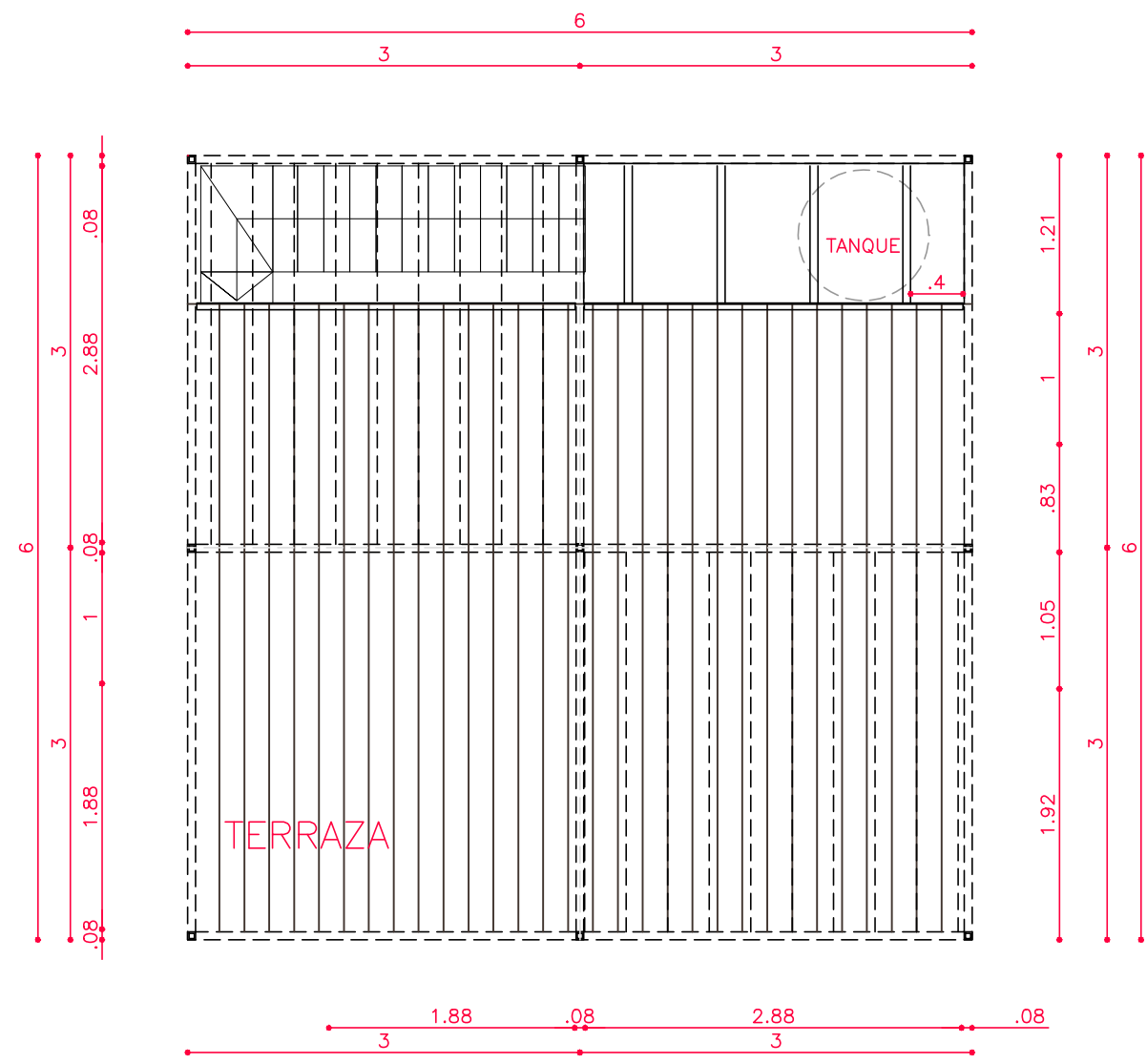
PLANTA ESTRUCTURA CUBIERTA
