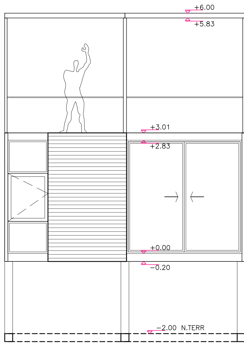
VISTA SUDOESTE
