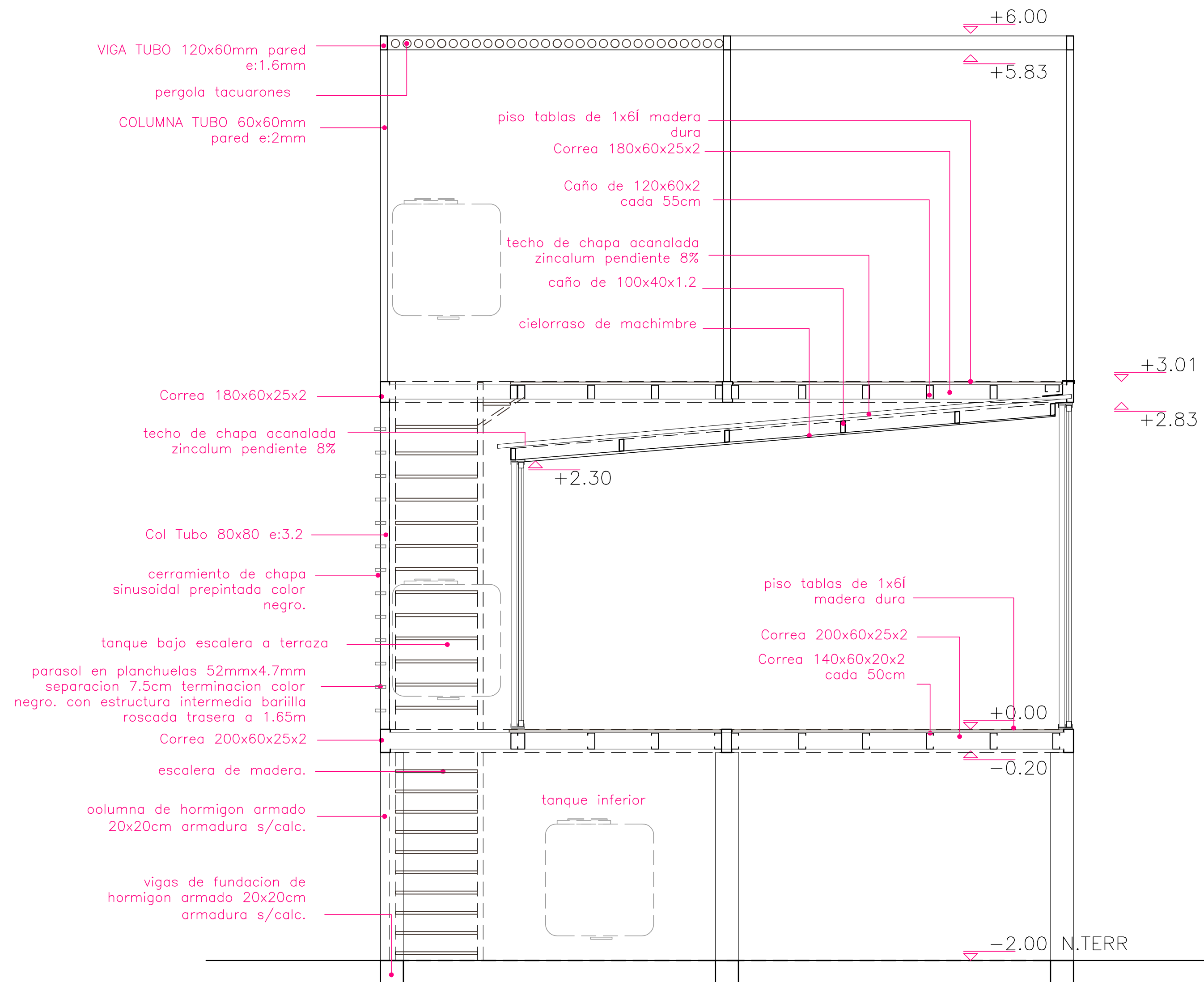
CORTE COMEDOR ESTAR
