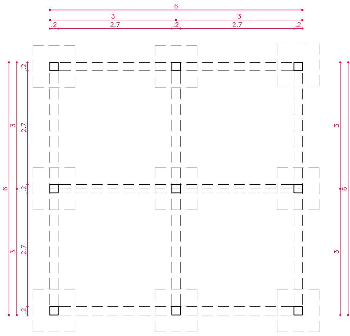
PLANTA ESTRUCTURA DE FUNDACION
