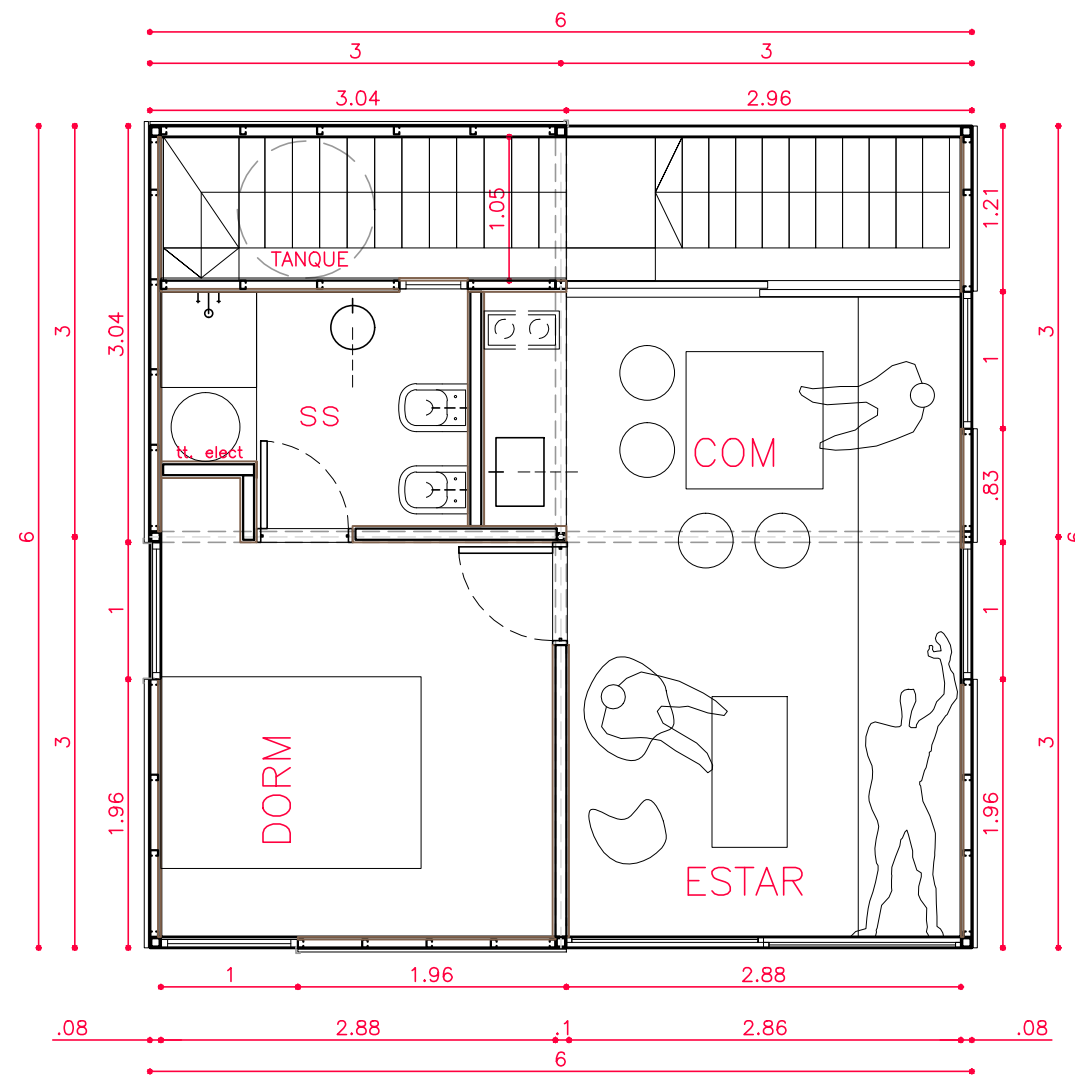
PLANTA ARQUITECTURA
