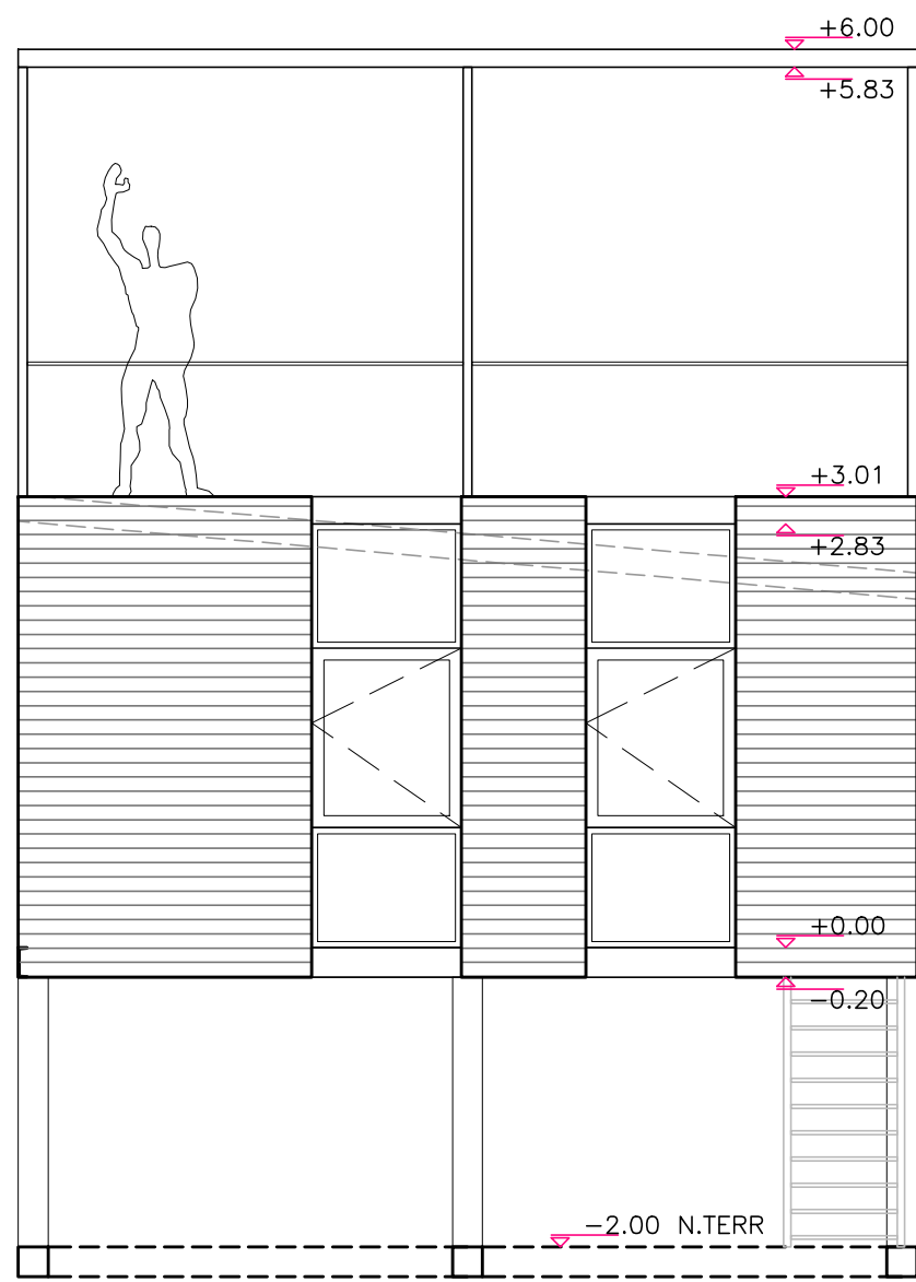
VISTA SUDESTE
