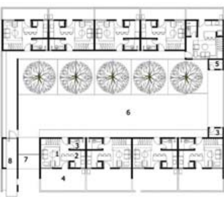
PLANTA 1o. PAVIMENTO
